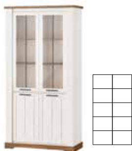
COUNTRY 12 | witryna 4-drzwiowa | 4 door display unit opcjonalne oświetlenie | optional lighting szer. x wys. x gł. | W x H x D 104 x 204 x 45 cm
